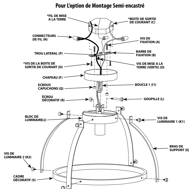
FIGURE 2. Il est possible que le dessin illustré ici ne soit pas la reproduction exacte de l'appareil d'éclairage contenu dans la boîte. Les instructions d'installation demeurent cependant valables.
