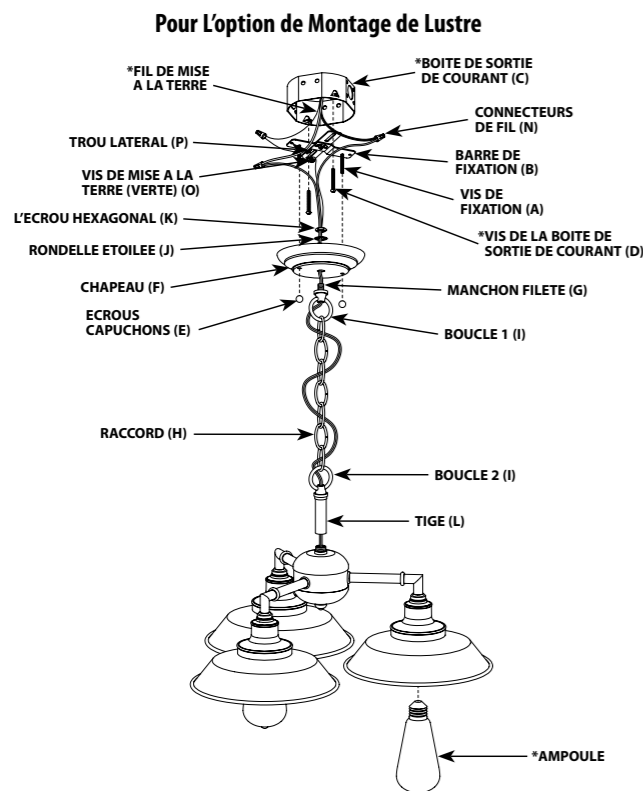
FIGURE 1. Il est possible que le dessin illustré ici ne soit pas la reproduction exacte de l'appareil d'éclairage contenu dans la boîte. Les instructions d'installation demeurent cependant valables.
