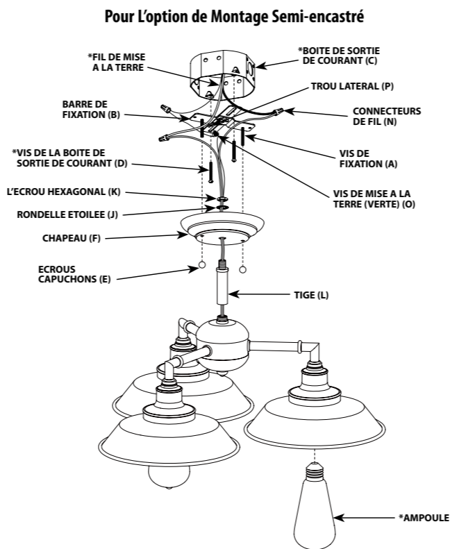
FIGURE 2. Il est possible que le dessin illustré ici ne soit pas la reproduction exacte de l'appareil d'éclairage contenu dans la boîte. Les instructions d'installation demeurent cependant valables.
